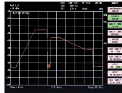
Actual waveform displayed on spectrum analyzer
